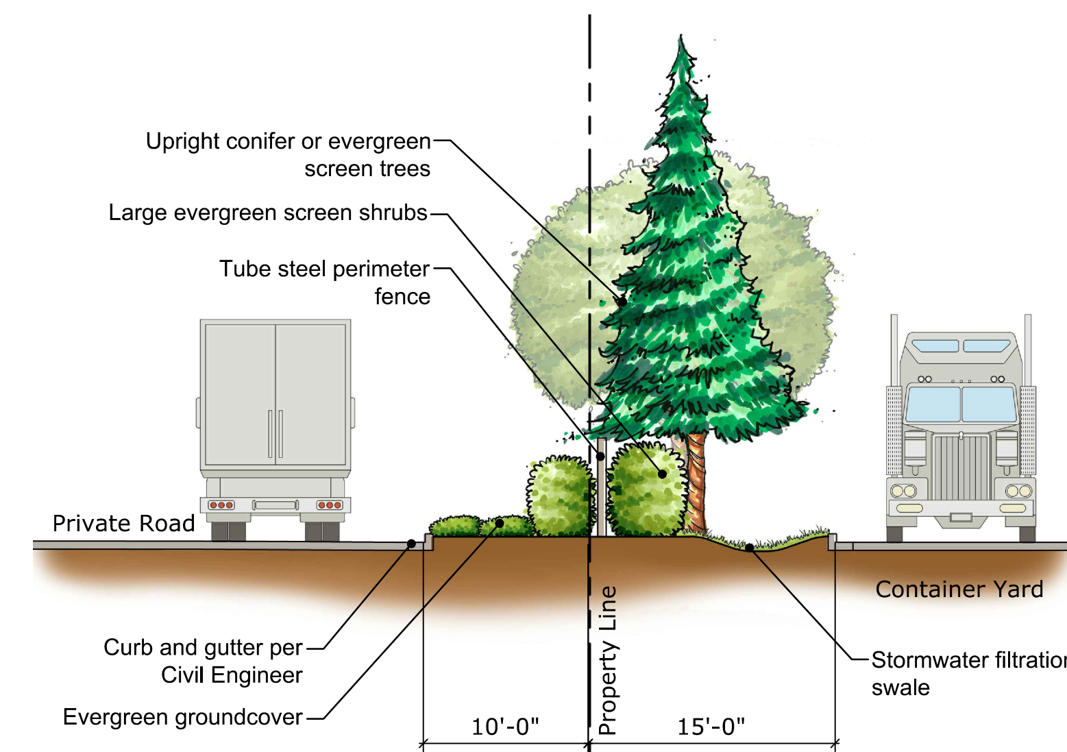
Section 'B'
