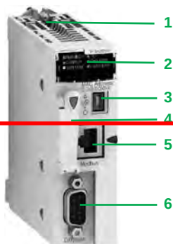
BMX P34 2010
