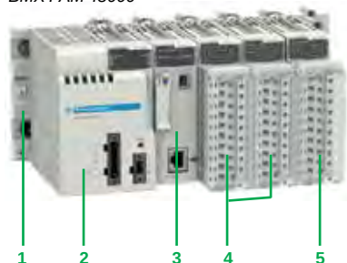
BMX PAM 48000
