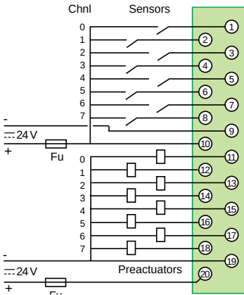
BMX DDM 16022
