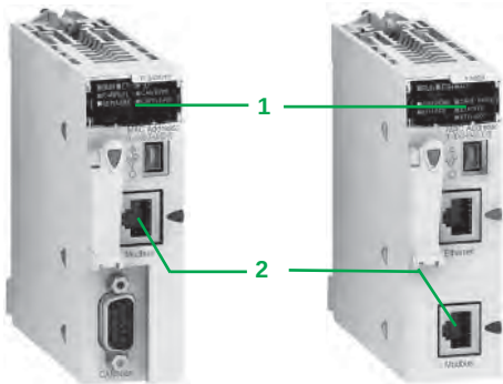
BMX P34 20102
