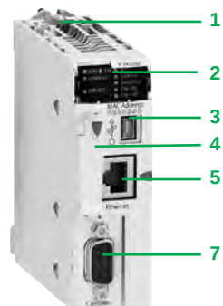
BMX P34 2030
