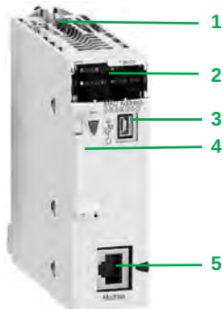
BMX P34 1000
